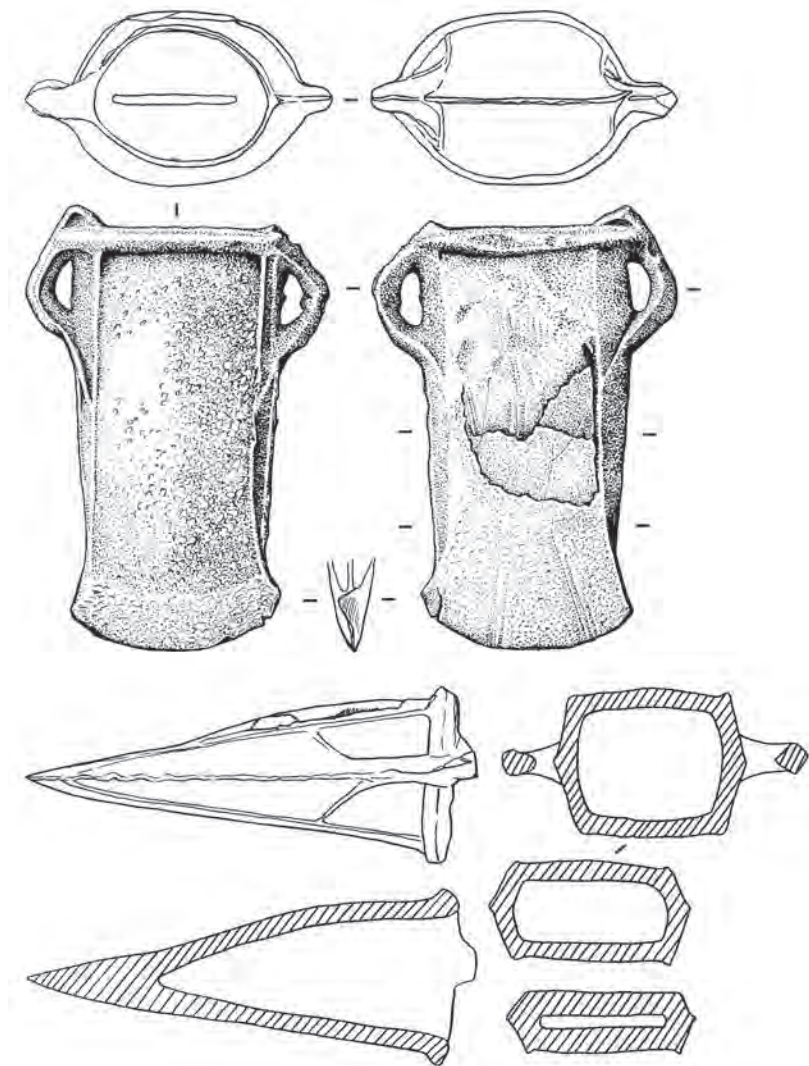
Рис. 2. Бронзовый кельт (детальная иллюстрация)
