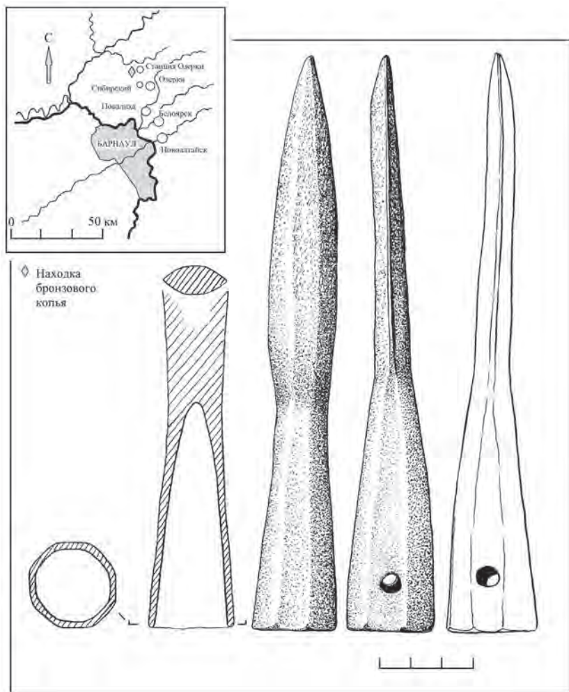
Рис. 1. Бронзовое копье из с. Станция Озерки
