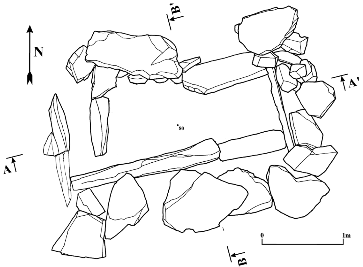
Рис. 8. Усть-Каменка-II, курган №2. Каменный ящик и первая насыпь. План
