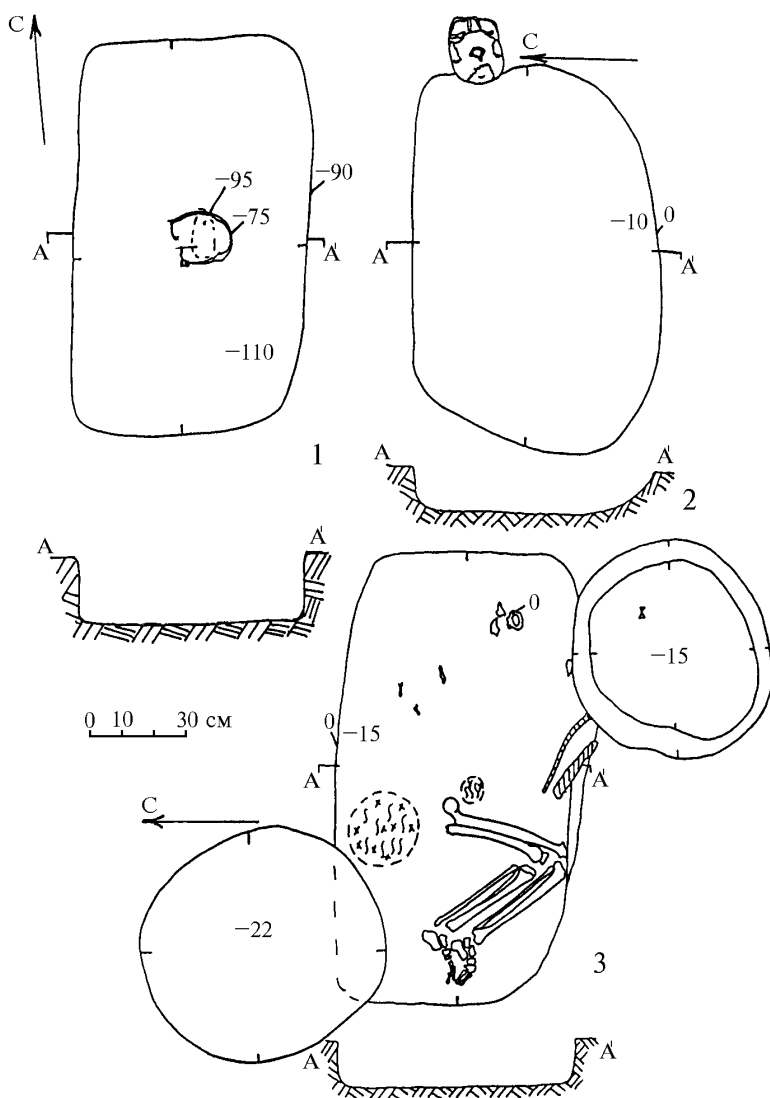
Рис. 31. Телеутский Взвоз-I: 1 — могила №22; 2 — могила №25; 3 — могила №23. Планы и разрезы
